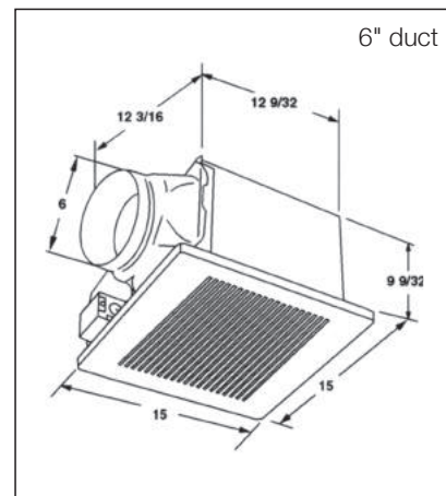
FV-30VQ3
